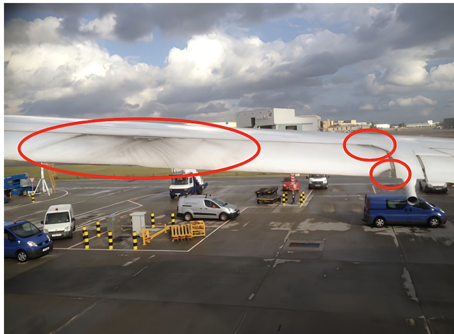
Punaiset ympäröidyt alueet ovat Unitedin 787 salamien kiinnittymispisteet oikeassa siivessä. Kuva: NTSB.
