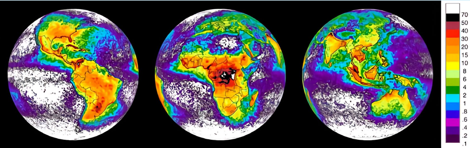
Salamoiden maailmanlaajuinen jakautuminen vuosina 1995–2003; väriskaala kuvaa keskimääräistä vuotuista salamojen lukumäärää neliökilometriä kohti. Kuva: Yhdysvaltain meri- ja ilmakehävirasto (NOAA) ja Yhdysvaltain ilmailu- ja avaruushallinto (NASA).
